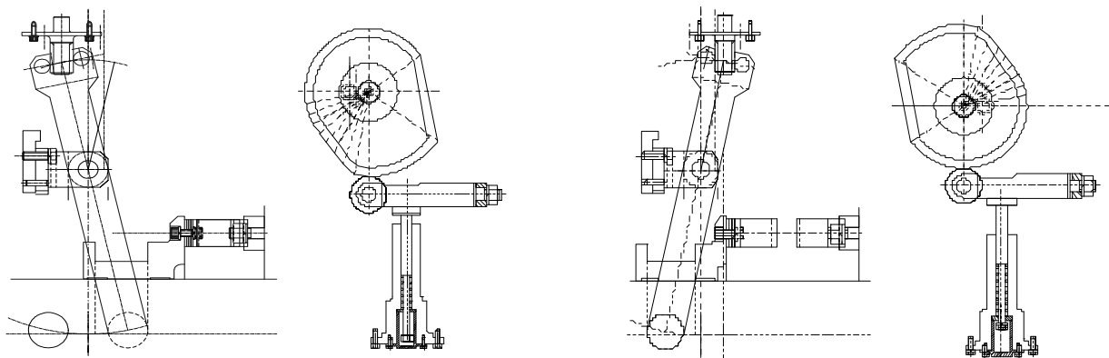
Figura 4.22. – Escovas levantadas.
