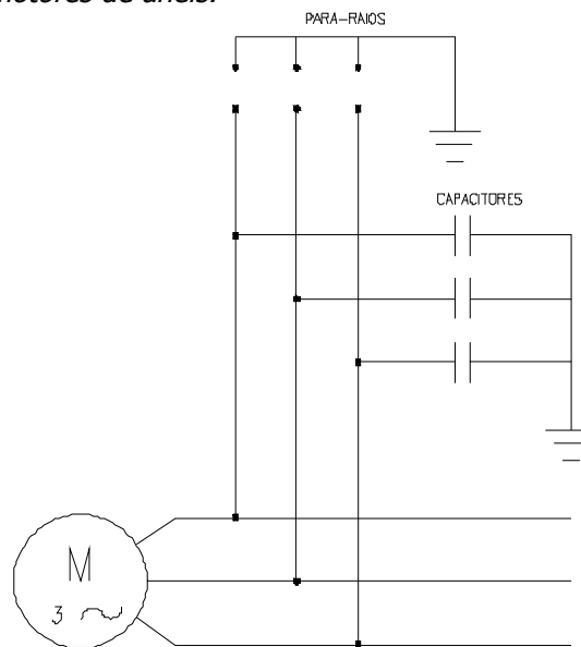
Figura 3.17 - Esquema de ligação geral para motores de anéis.
