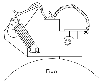
Figura 4.9 – Escova para aterramento do eixo.
