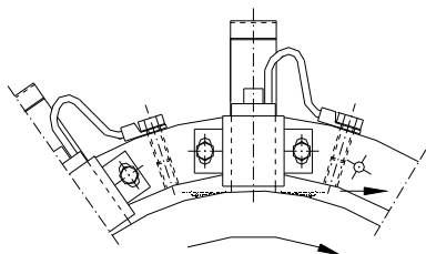
Figura 4.8 - Assentamento das escovas.
