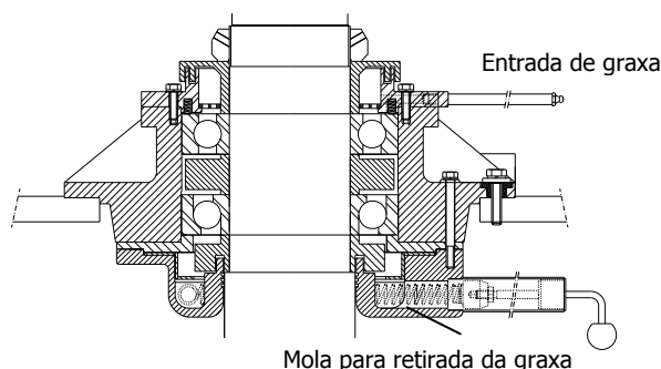
Figura 4.3. - Exemplo de um mancal de rolamento traseiro vertical com saída de graxa com dispositivo de mola.
