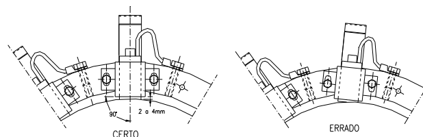
Figura 4.6 – Montagem do porta-escovas.
