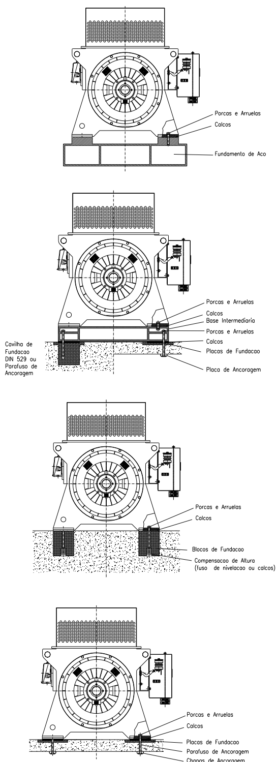
Figura 3.2 - Forma de fixação de motores.
