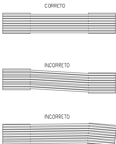
Figura 3.11 - Correto alinhamento das polias. A tensão na correia deverá ser apenas suficiente para evitar o escorregamento no funcionamento (figura 3.12).
