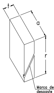
Figura 4.7 - Marca de desgaste da escova.
