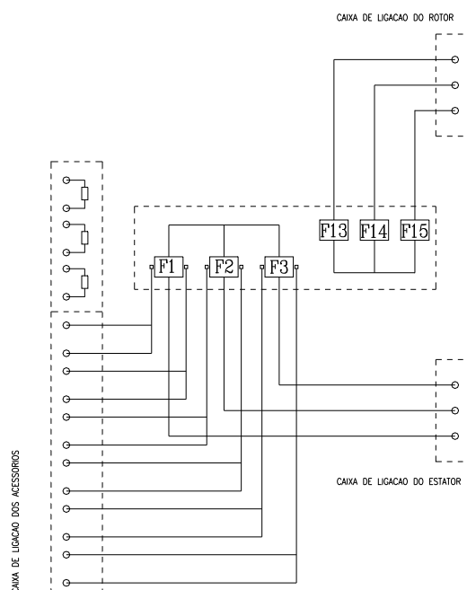
Figura 3.17 - Esquema de ligação geral para motores de anéis.
