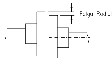
Figura 3.6b - Desvio de concentricidade.
