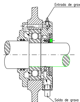
Fig. 4.2. - Rolamentos e sistemas de lubrificação.
