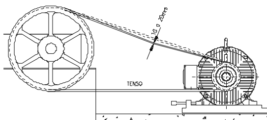
Figura 3.12 - Tensões na correia.
