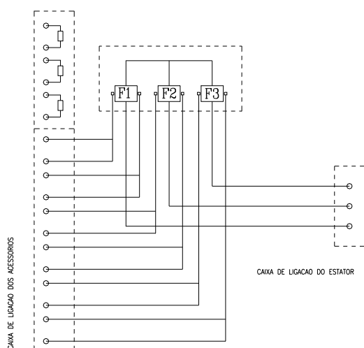
Figura 3.16. - Esquema de ligação geral para motores de gaiola.
